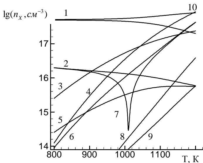
Рис.2. Залежність концентрації носіїв струму і точкових дефектів у CdTe:In від температури відпалу: 1 – [A_{In}^-] ; 2 – n ; 3 – [Te_i^-] ; 4 – [V_{Cd}^-] ; 5 – [V_{Cd}^{2-}] ; 6 – p ; 7 – N_x ; 8 – [Cd_i^{2+}] ; 9 – [V_{Te}^{2+}] ; 10 – [In_{Cd}^+] . Концентрація індію In_{tot} = 10^{18} \text{ см}^{-3} , парціальний тиск пари кадмію P_{Cd} = 10 \text{ Па} .
