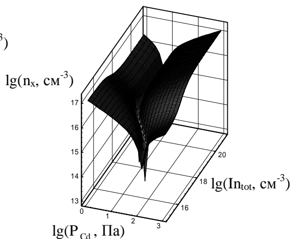
Рис.8. Розрахункова просторова фазова n_x - P_{Cd} - In_{tot} -діаграма рівноваги CdTe:In ( T = 1000\text{K} ).
