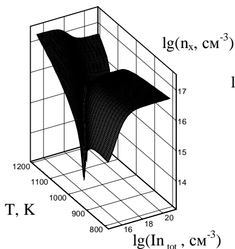
Рис.7. Розрахункова просторова фазова n_x - In_{tot} - T -діаграма рівноваги CdTe:In ( P_{Cd} = 50 \text{ Па} ).
