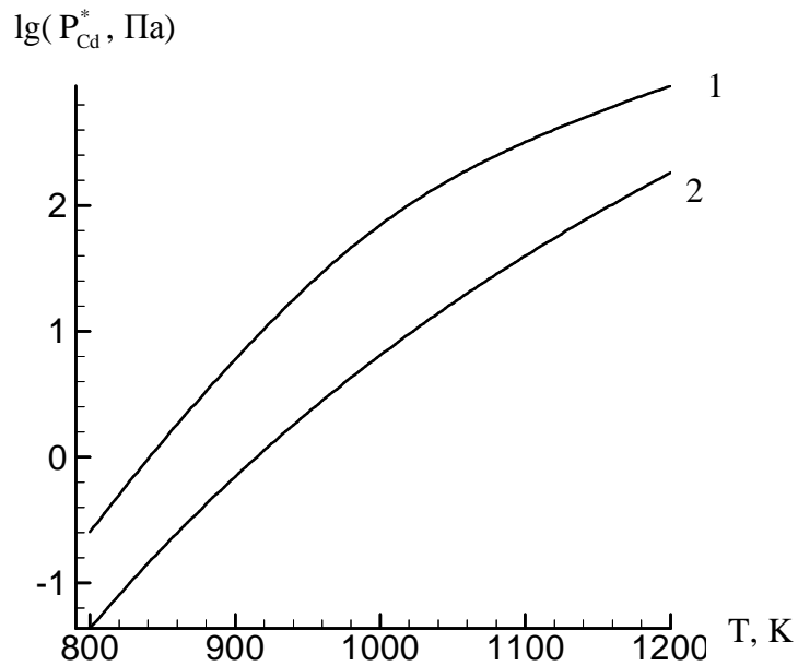
Рис.3. Залежність тиску пари кадмію, що відповідає термодинамічному n-p -переходу, у кристалах CdTe:In від температури відпалу при різних концентраціях індію In_{tot} , см^{-3} : 1 – 10^{16} ; 2 – 10^{18} .
