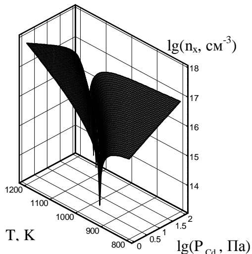
Рис.6. Розрахункова просторова фазова n_x - P_{Cd} - T -діаграма рівноваги CdTe:In ( In_{tot} = 10^{20} \text{ cm}^{-3} ).
