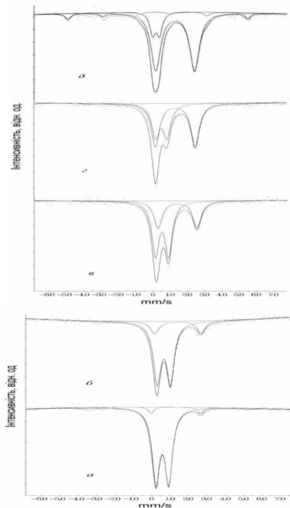
Рис. 2. Гамма-резонансні спектри поглинання, отримані від нанодисперсного \text{TiO}_2\langle 20\% \text{Fe}\rangle , інтеркальованого іонами \text{Li}^+ , при різних значеннях “гостьового” навантаження: а) x = 0,17 ; б) x = 0,5 ; в) x = 0,8 ; г) x = 1,1 ; д) x = 1,75 .
