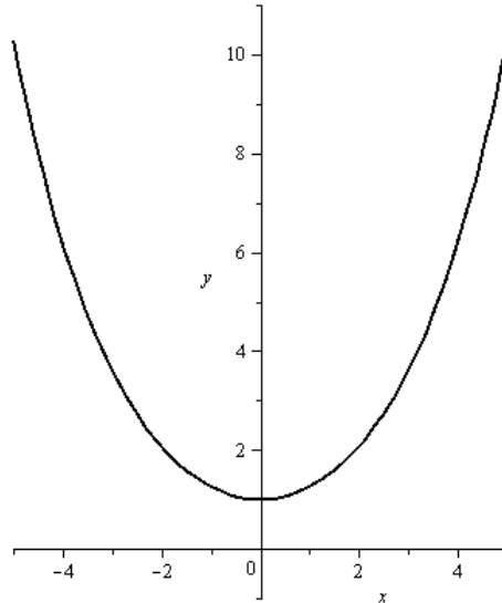
Рисунок 2 – Графік функцій y = \text{Chc}(x)
