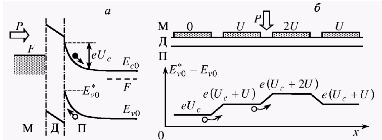
прилади із зарядовим зв'язком
