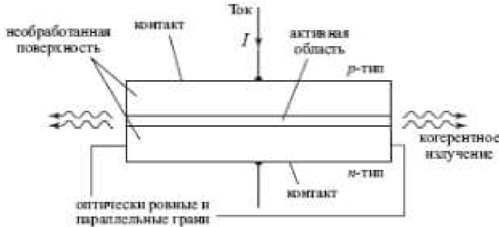
Інжекційний лазер - схема
