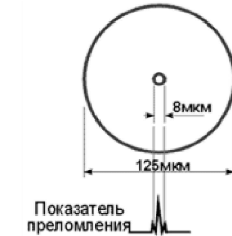
зі зміщеною дисперсією (DSF)
