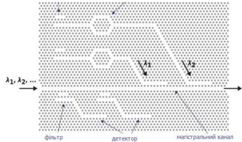
Рис. 4. Фільтрація хвиль структурою на основі фотонного кристала
