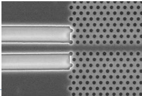
Рис. 3. Підведення інтегрального хвилеводу до ФК
