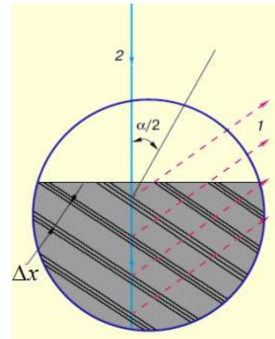
Схема інтерференції при зчитуванні
