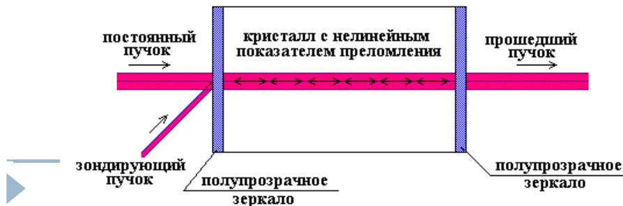
Интерферометр Фабри-Перо
