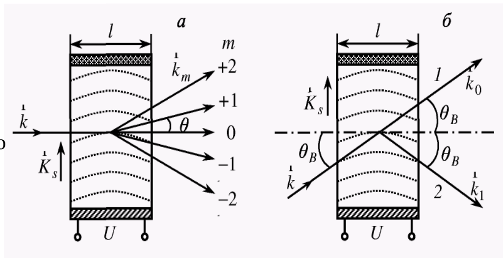
Дифракція світла на ультразвукових хвилях в режимах Рамана - Ната (а) і Брега (б)
