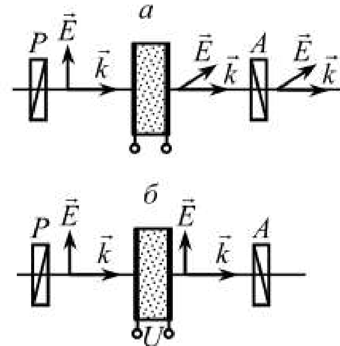
Схема спостереження твіст - ефекту: а - просвітлений стан РК-комірки ( U = 0 ); б - затемнений стан РК-комірки ( U \neq 0 )
