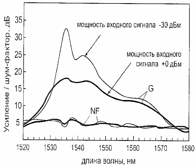
Спектральна залежність коефіцієнта шуму та підсилення ербієвого підсилювача
