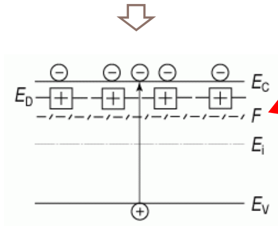
Зонна діаграма напівпровідника n-типу
