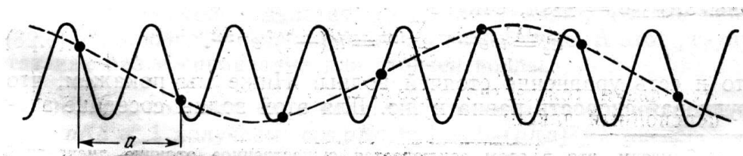
Майже вільні електрони
