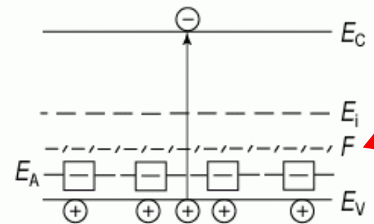
Зонна діаграма напівпровідника p-типу
