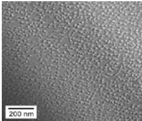
Двомірний масив квантових точок
