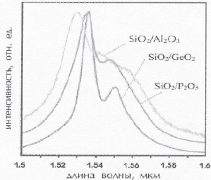
Спектри випромінювання іонів ербію в кварцевому склі з різними добавками
