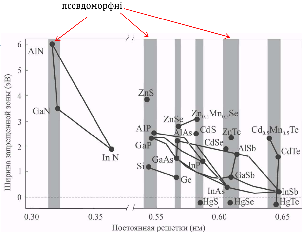
Матеріали, що використовуються при формуванні надґраток
