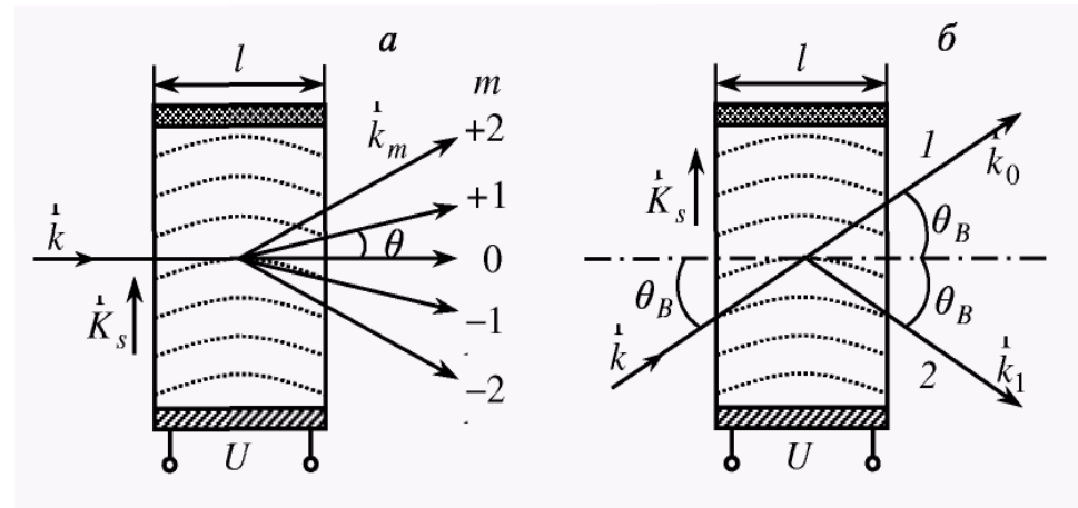
Дифракция света на ультразвуковых волнах в режимах Рамана - Ната (а) и Брегга (б)
