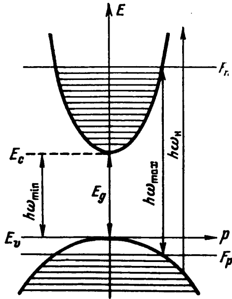
Інверсна заселеність в прямозонному напівпровіднику
