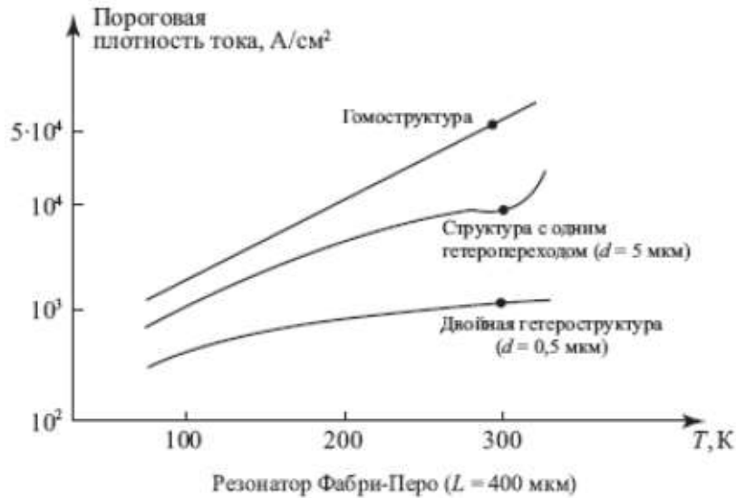
Умова лазерної генерації
