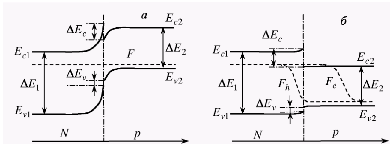
Зонна діаграма різкого N-p-гетеропереходу в стані термодинамічної рівноваги (а) і при прямому зсуві (б)
