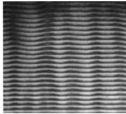
Тримірний масив квантових точок
