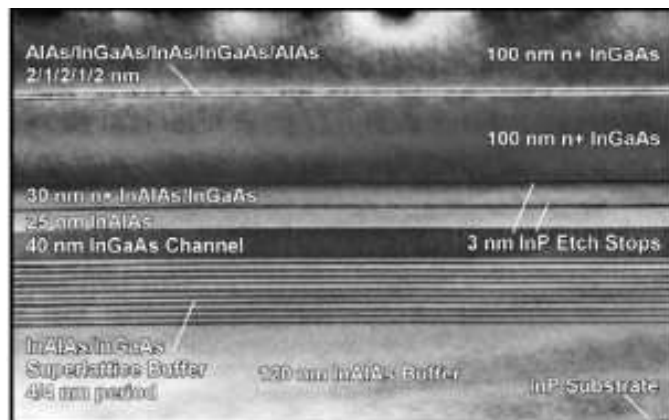
Багатошаровий масив квантових ям
