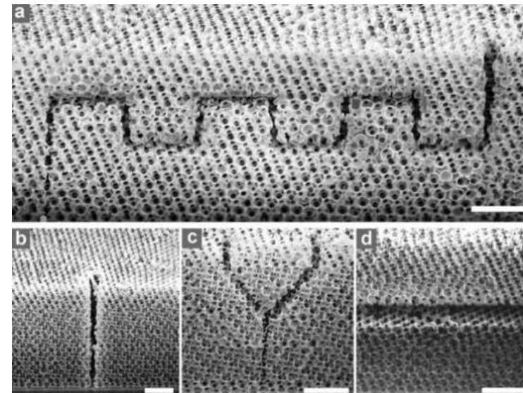
Рис. 5. Канали ФК, вигравлені методом двофотонної полімеризації
