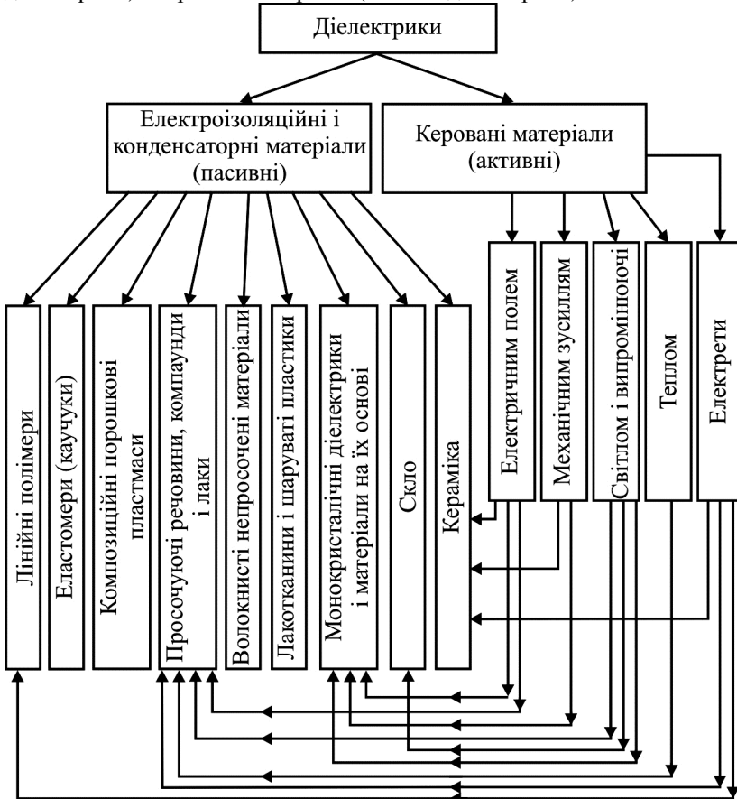
Рис. 3.1. Класифікація діелектриків
