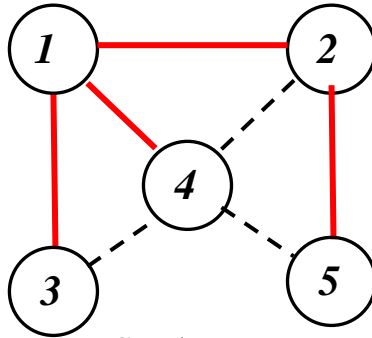
Рисунок 11.4 – Результат BFS-обходу, починаючи з вершини v_1
