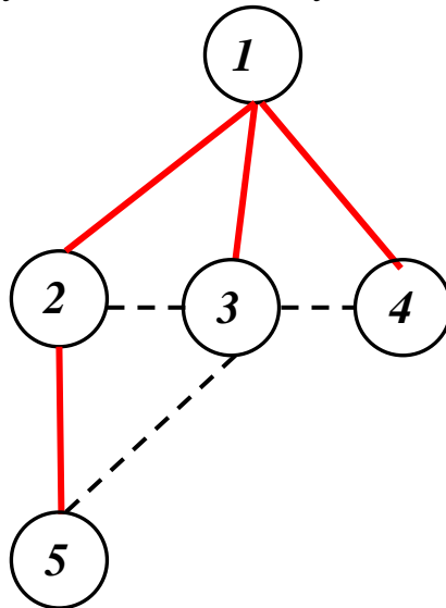
Рисунок 11.4 – Результат BFS-обходу, починаючи з вершини v_1
