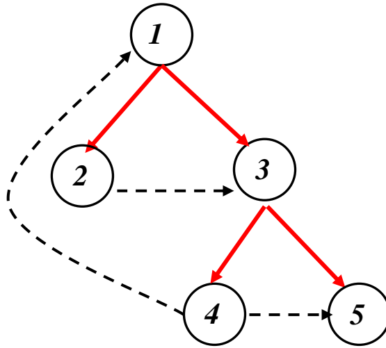
Рисунок 11.10 – Результат BFS-обходу, починаючи з вершини v_1
