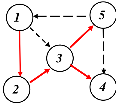
Рисунок 11.7 – Результат DFS-обходу, починаючи з вершини v_1
