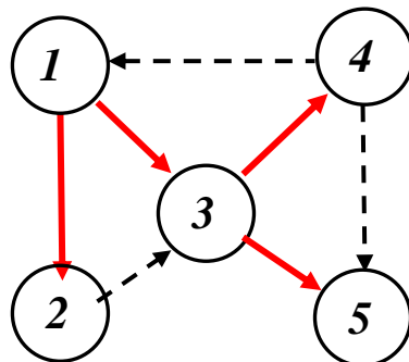
Рисунок 11.9 – Результат BFS-обходу, починаючи з вершини v_1
