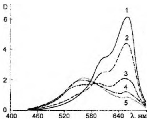
Рис. 1. Спектри системи полістиренсульфонат-метиленовий синій, співвідношення ПСС:МВ: 1 – 0,0; 2 – 0,17; 3 – 0,52; 4 – 0,69; 5 – 1,12.
