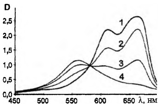
Рис. 4. Спектри барвника метиленовий синій (1) і його комплексу з карагінаном (2), (3), (4): вміст карагінану (0,6-2,0) \cdot 10^{-3}\% .
