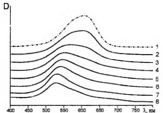
Рис. 7. Спектри поглинання BV41, сорбованого на бентоніті за кількістю барвника в системі (ммоль на 100 г глини): 1 – 0; 2 – 333,3; 3 – 166; 4 – 125; 5 – 100; 6 – 90; 7 – 40; 8 – 16,6.
