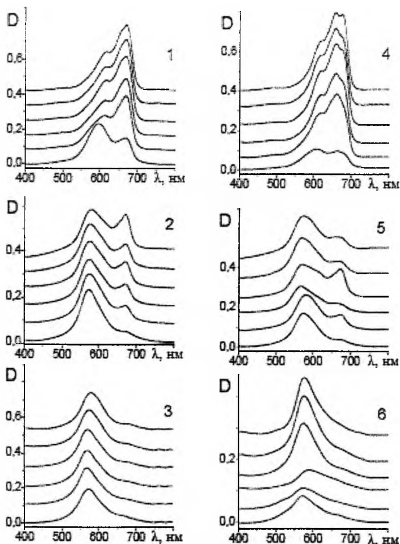
Рис. 5. Спектри свіжоприготовлених дисперсій (1, 2, 3) та дисперсій після 18 год. старіння (4, 5, 6) Lap (1, 4), Kun (2, 5) та FH (3, 6) з барвником метиленовим синім.
