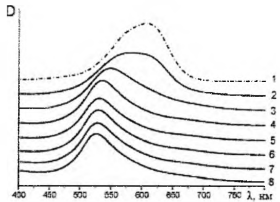
Рис. 6. Спектри поглинання BV41, сорбованого на монтморилоніті за кількістю барвника в системі (ммоль на 100 г глини): 1 – 0; 2 – 333,3; 3 – 166; 4 – 125; 5 – 100; 6 – 90; 7 – 40; 8 – 16,6.
