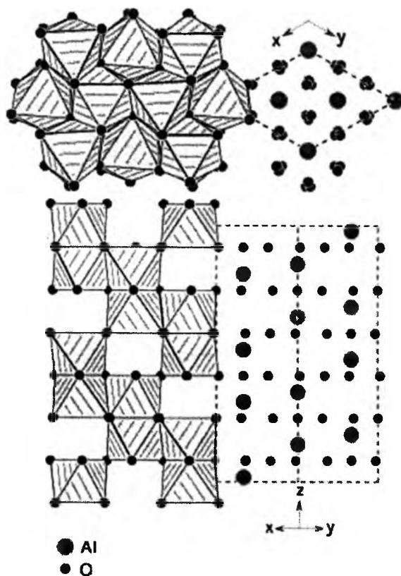
Рис. 1. Ромбоєдрична кристалічна структура \alpha\text{-Al}_2\text{O}_3 (просторова група R\bar{3}c ). Пари сполучених по гранях октаєдрів проходять уздовж осі третього порядку. Видно двовимірні нескінченні шари конденсованих октаєдрів. Внизу показано проекцію такого шару вздовж напрямку [110] .
