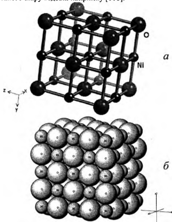
Рис. 2. Кубічна структура нікол(II) оксиду (структурний тип натрій хлориду): а – стерженькульова модель; б – щільноупакована структура ( \text{Ni-O-Ni} = 0,41684 \text{ nm} ).
