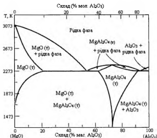
Рис. 1. Фазова діаграма системи MgO - Al_2O_3 [12].
